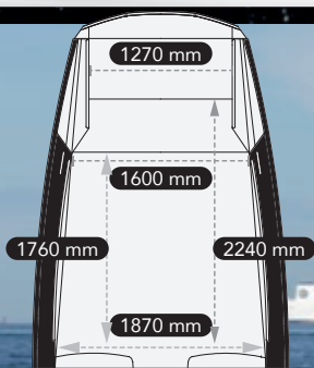
Keulan mitat
