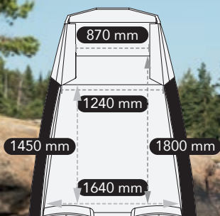
Keulan mitat
