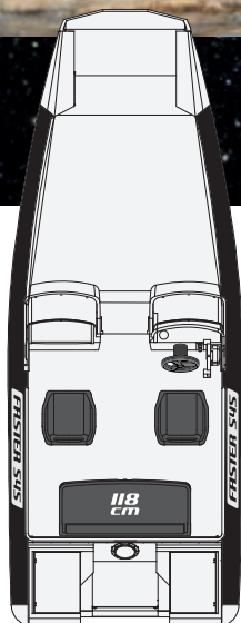
Keulan mitat
